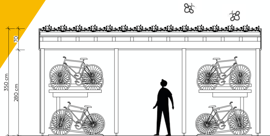
SCHNITT
